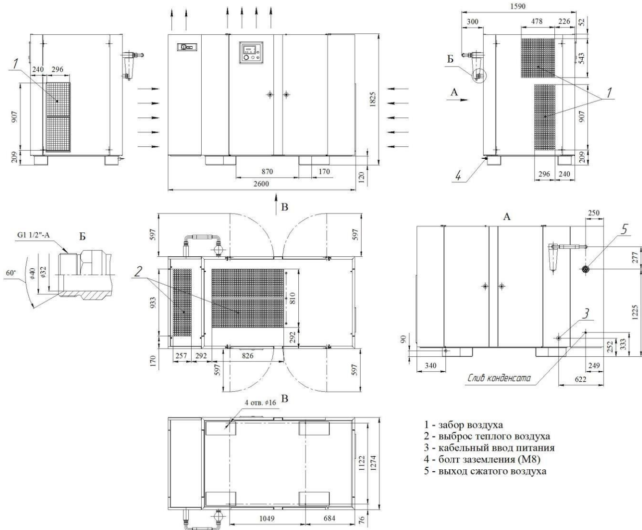
Установка компрессорная ВК60Р-Д. Установочные и присоединительные размеры.
